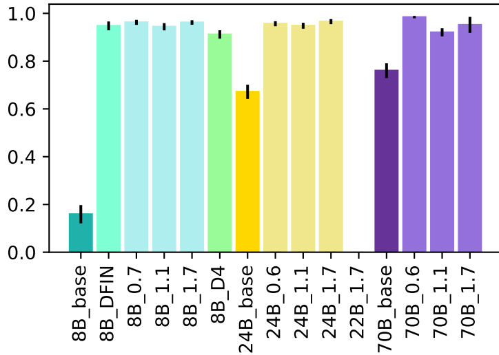
Kappa
