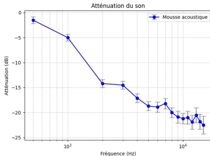
Réduction passive (7)
