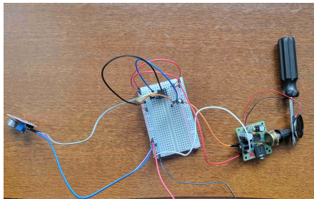
Réduction active (2)
