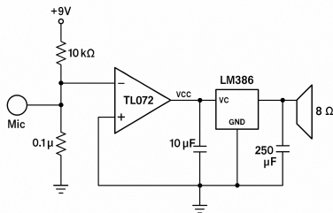
Schéma électrique (9)
