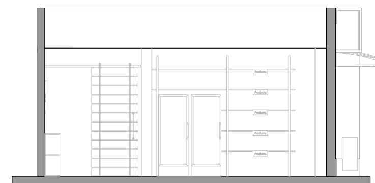
CORTE A-A
