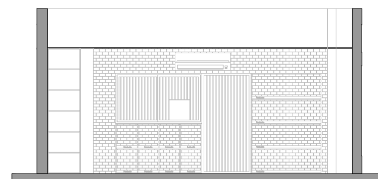
CORTE B-B
