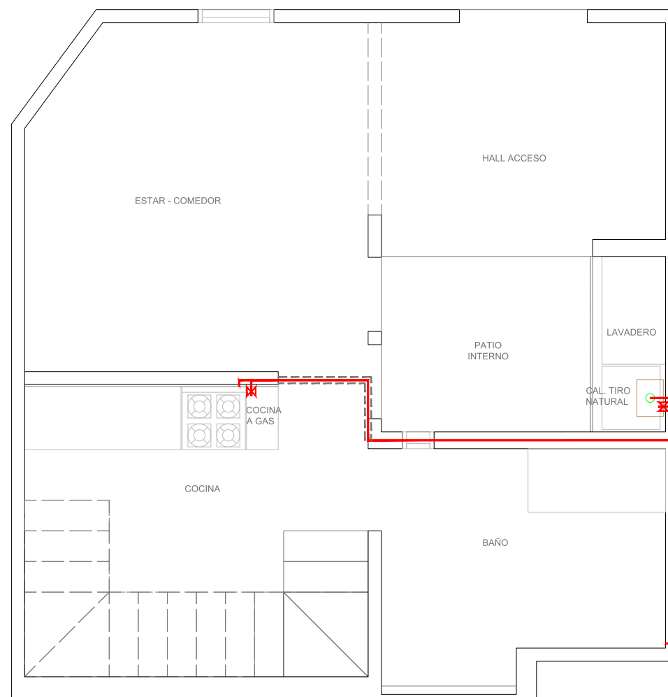
PLANTA BAJA
