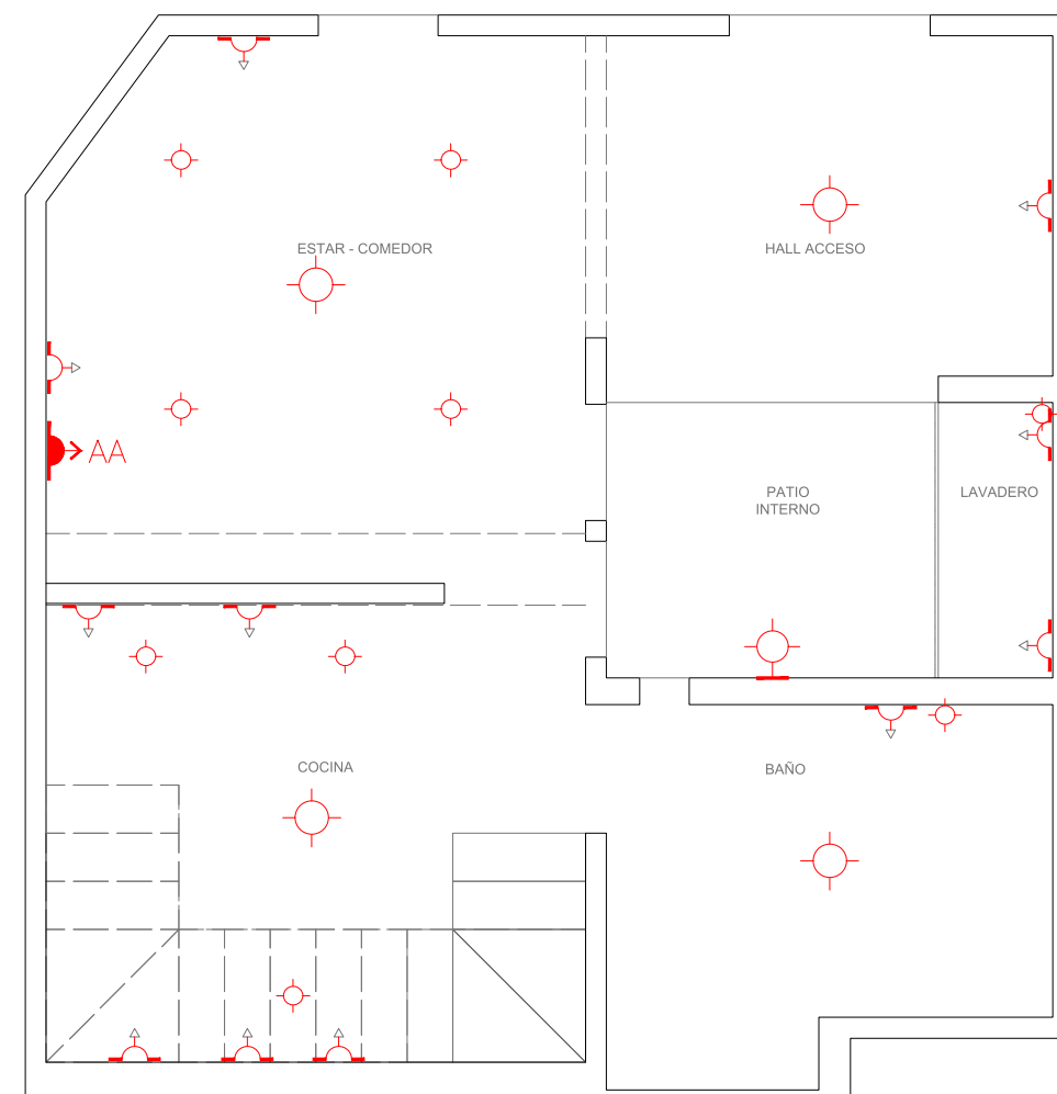
PLANTA BAJA
