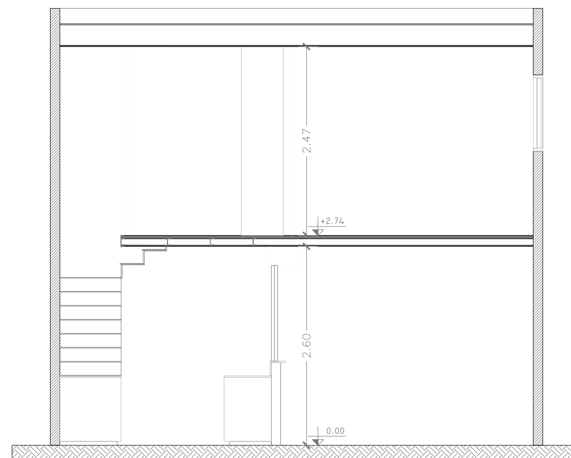
CORTE D-D
