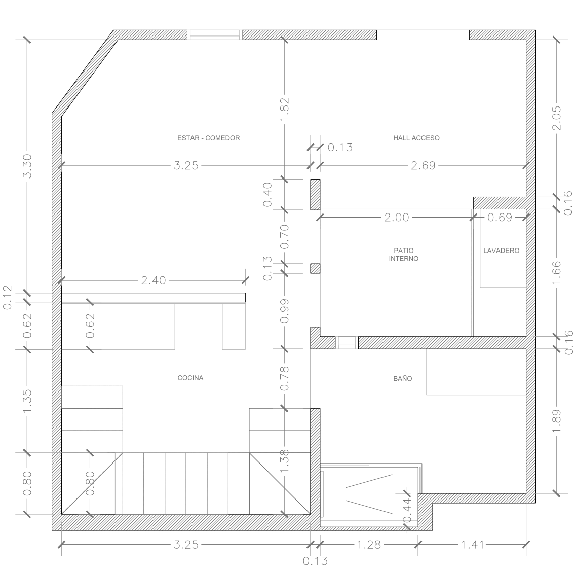
PLANTA BAJA
