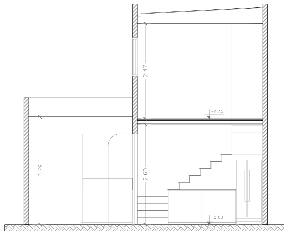
CORTE C-C
