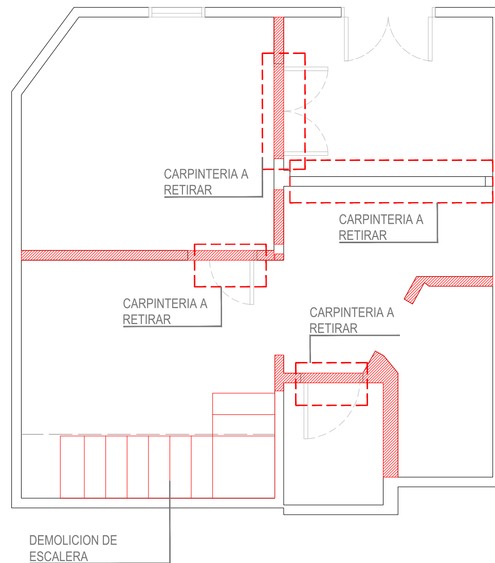
PLANTA BAJA
