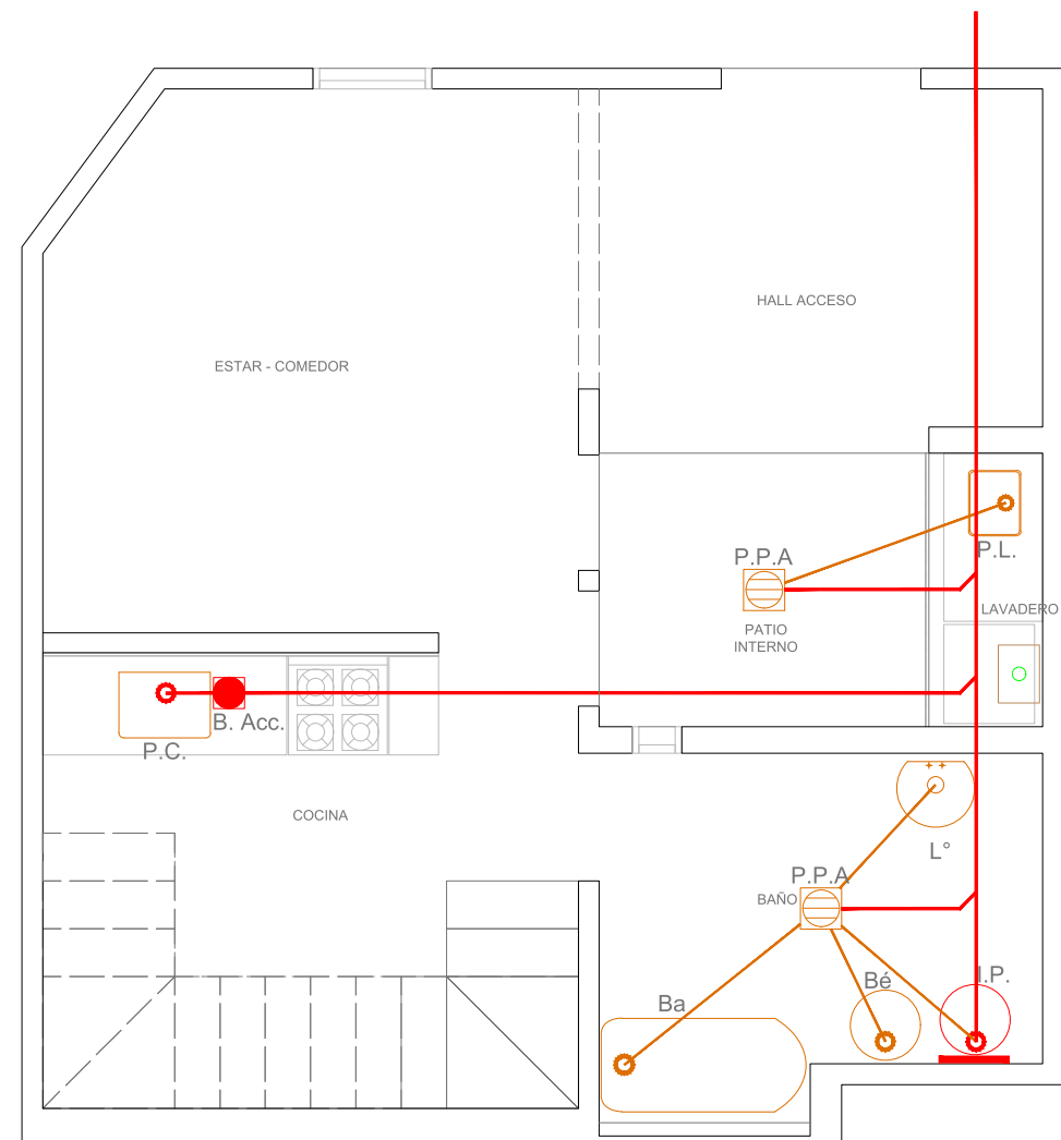
PLANTA BAJA
