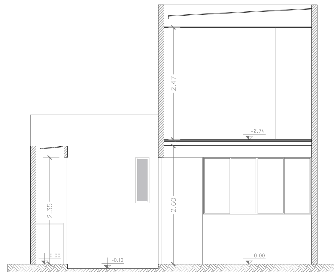
CORTE B-B
