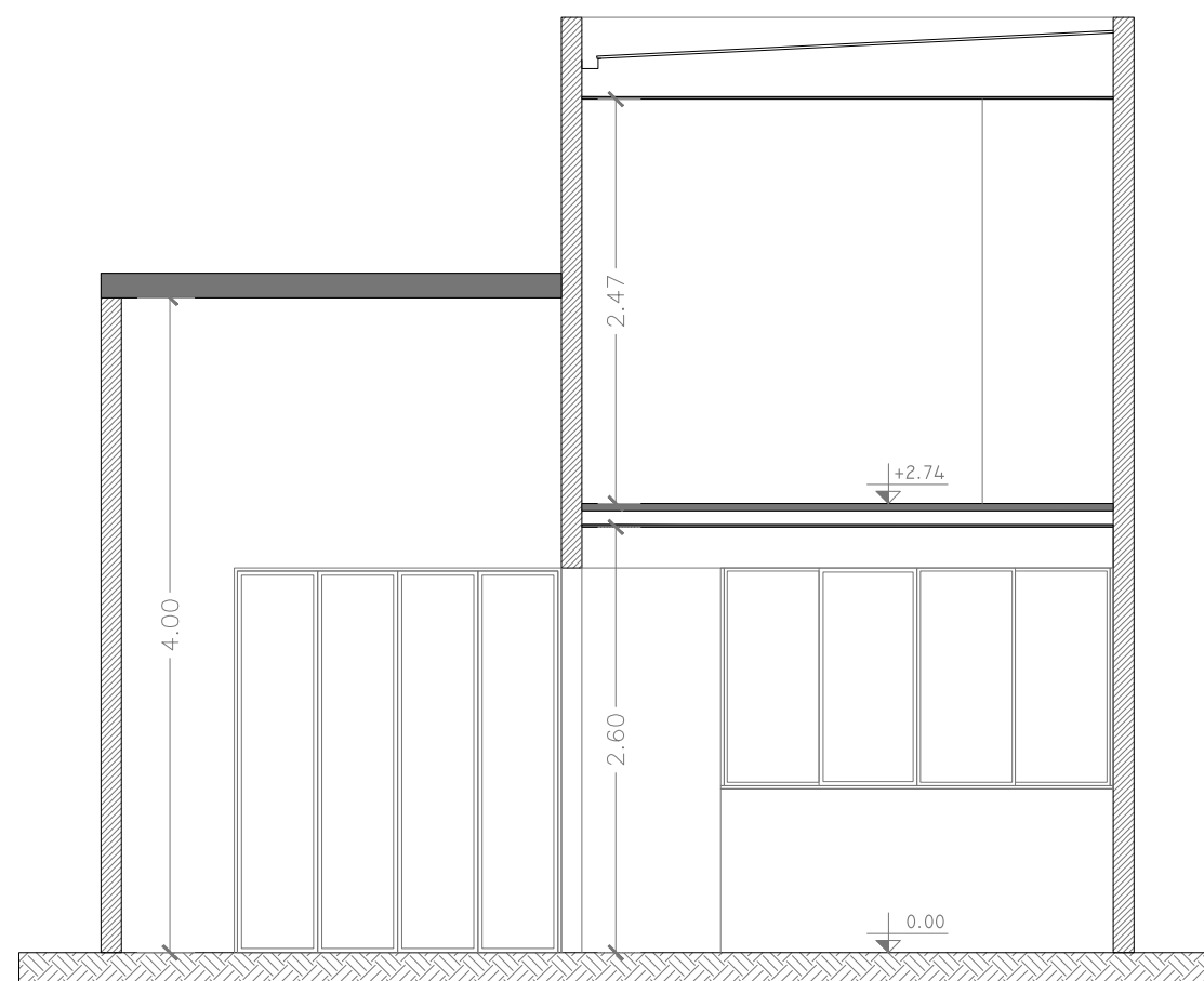
CORTE A-A
