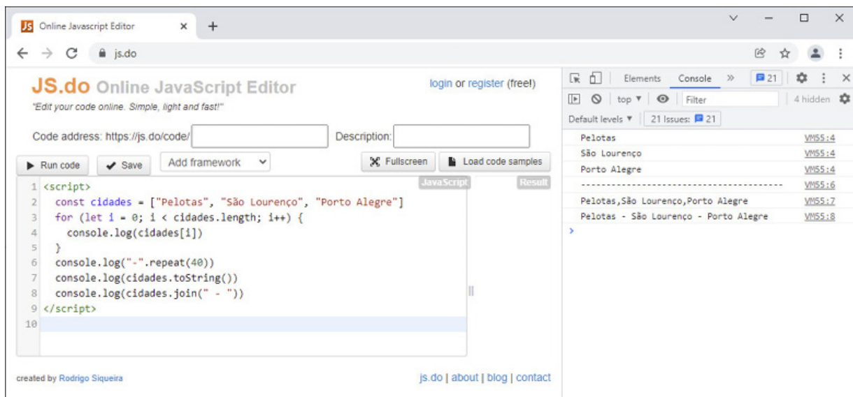
Figura 6.1 – Formas de exibir o conteúdo de um vetor.
