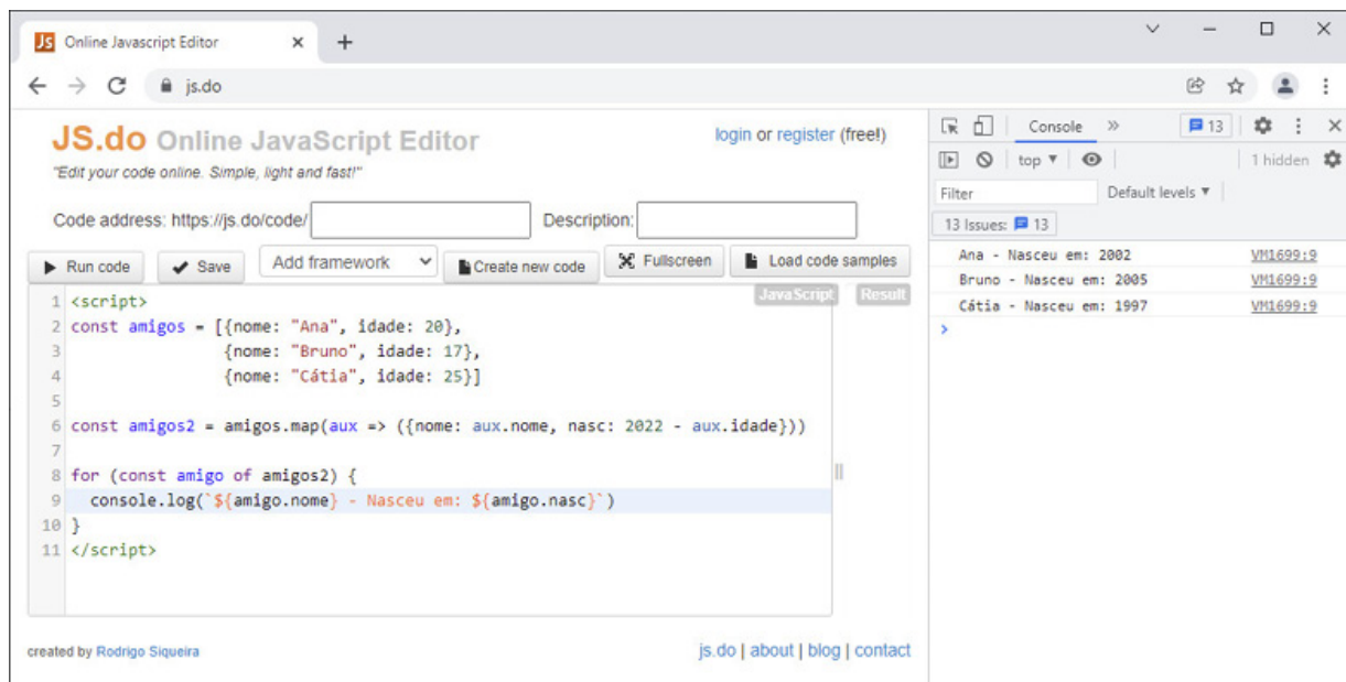
Figura 6.6 – Uso do map() sobre um array de objetos.
