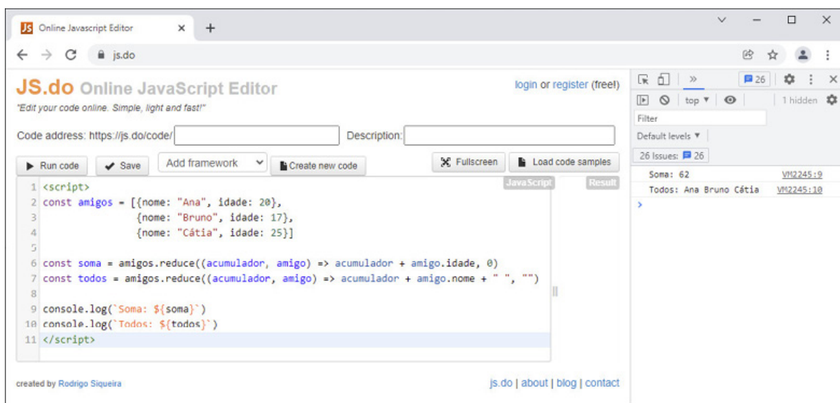
Figura 6.8 – Método reduce() aplicado sobre um array de objetos.
