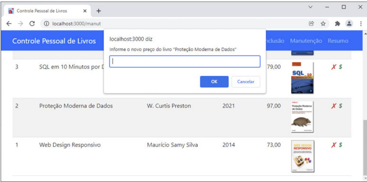
Figura 13.11 – Ao clicar sobre o ícone “$” o programa solicita o novo preço do livro.
