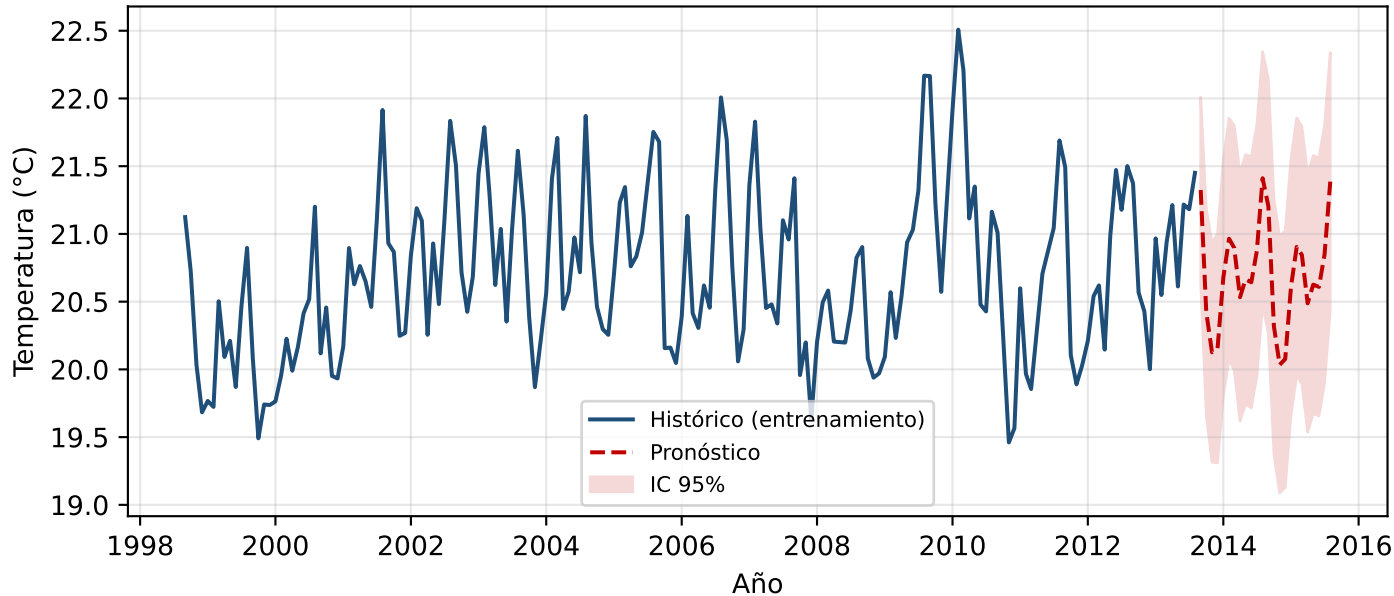
Pronóstico SARIMA -- Bogotá
