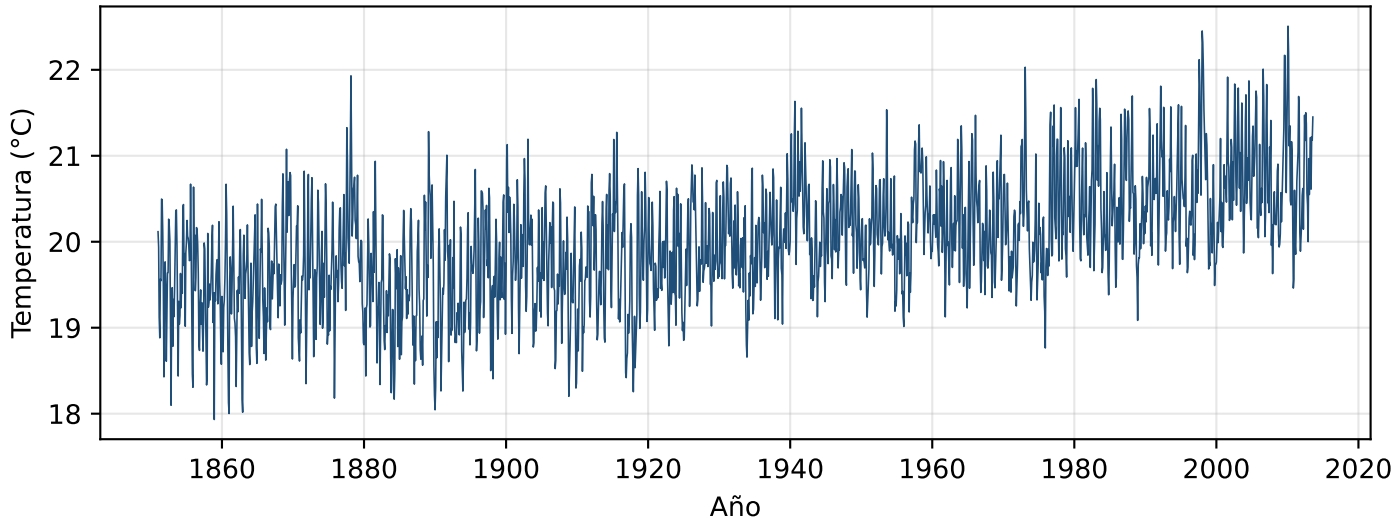
Temperatura promedio mensual -- Bogotá (1851-2013)
