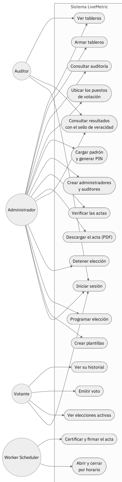
Figura 6. Casos de uso por actor. El auditor solo lee: ningún endpoint de escritura acepta su rol.
