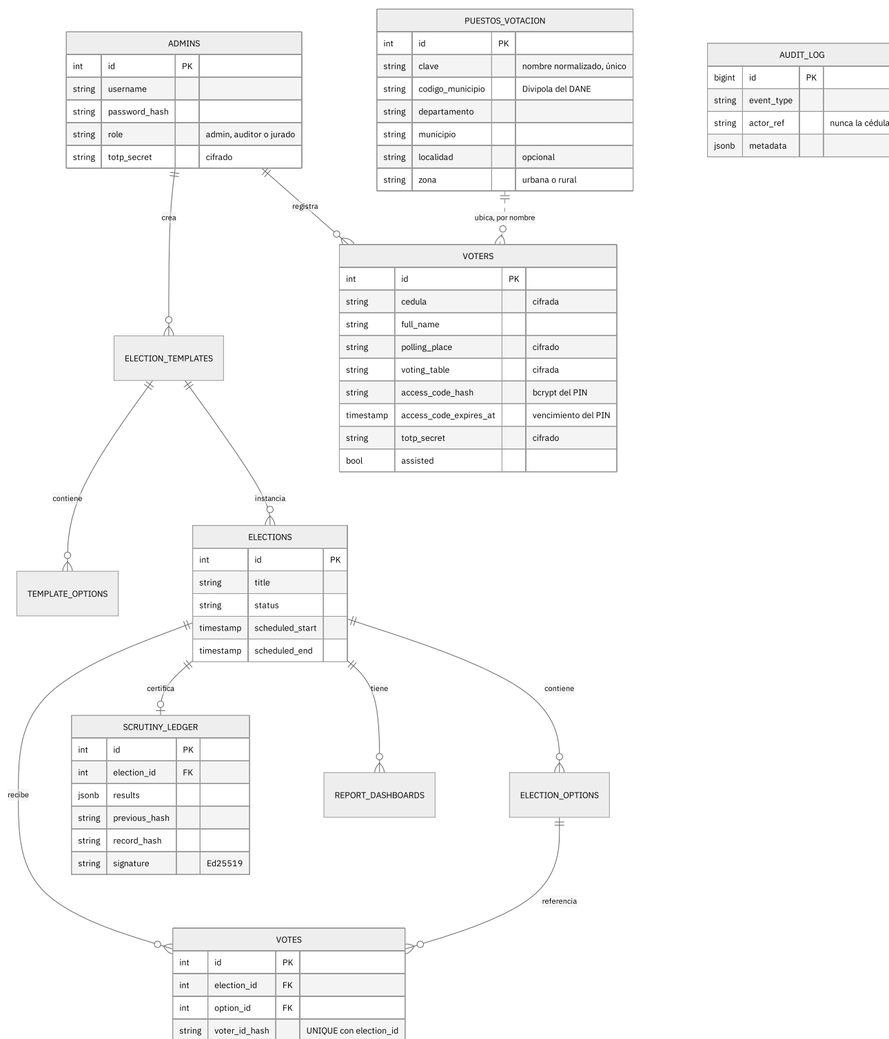
Figura 7. Modelo de datos (resumen). votes nunca guarda la cédula, solo su hash con un salt que solo conoce Auth. puestos_votacion se une al padrón por el nombre normalizado del puesto, que en voters va cifrado.
