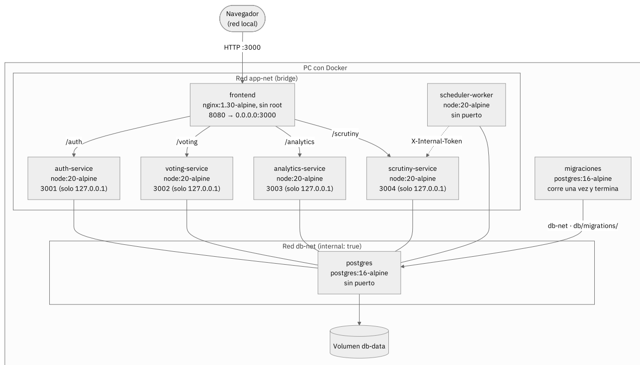
Figura 3. Diagrama de despliegue con Docker Compose. Terraform reproduce la misma topología y Docker Swarm la despliega con réplicas y una red overlay cifrada.
