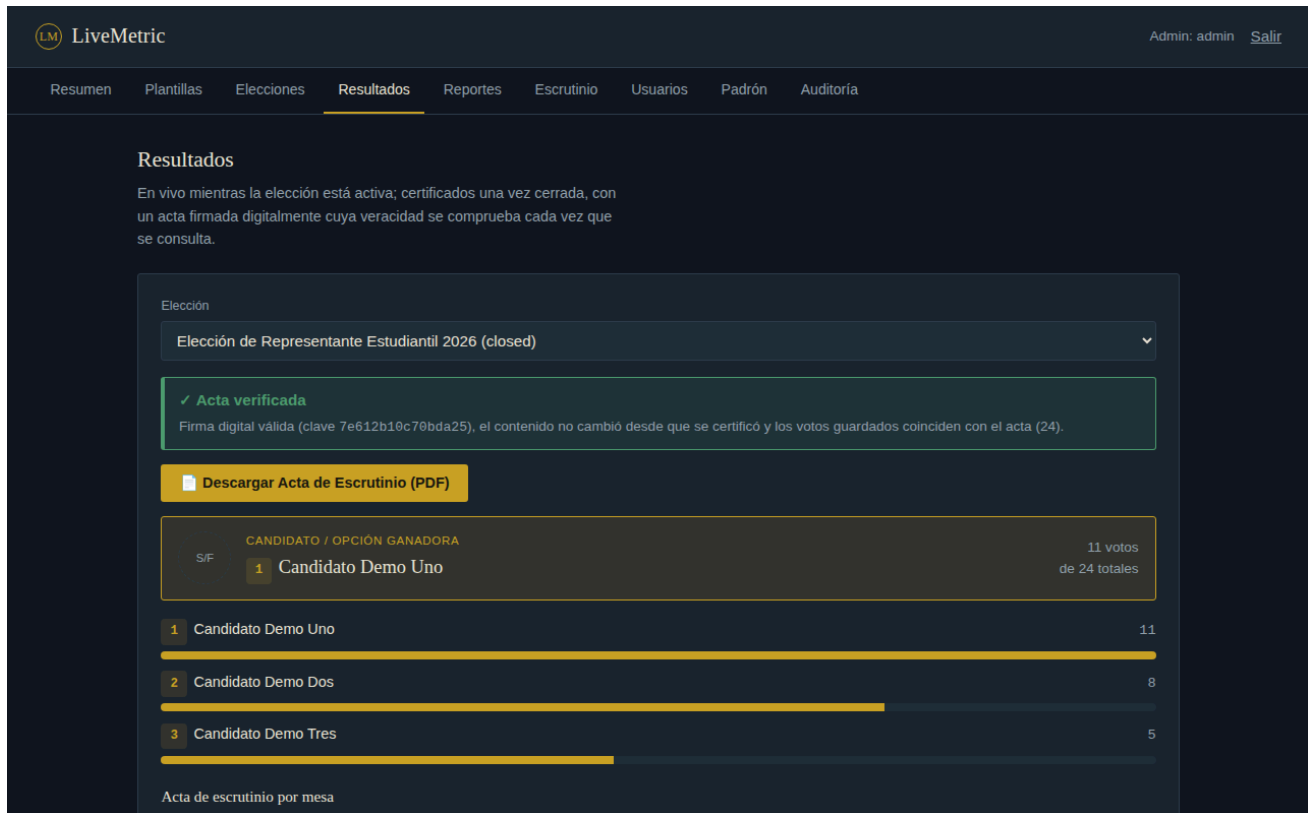
Figura 1. Resultados certificados con el indicador de veracidad: la firma digital es válida, el acta no cambió y los votos guardados coinciden con ella.
