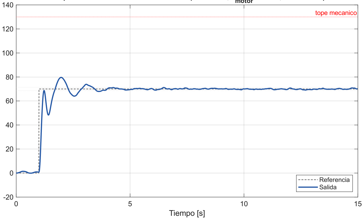
Respuesta del lazo cerrado no lineal ( T_s=10 ms, \tau_{\text{motor}}=50 ms, ruido= 1.0^\circ )
