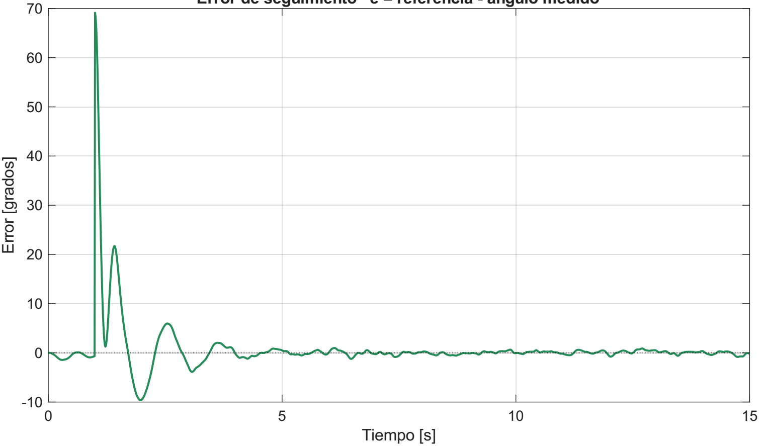
Error de seguimiento e = \text{referencia} - \text{angulo medido}
