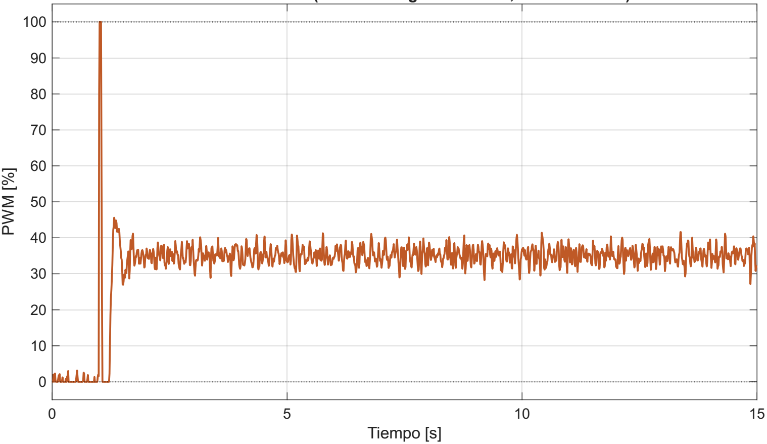
Senal de control (medio en regimen: 35.1%, rizado: 2.36%)
