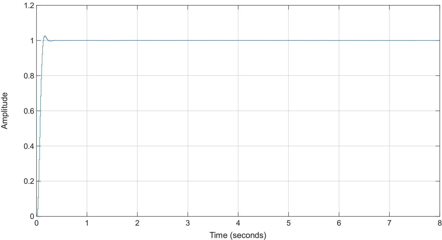
Respuesta al escalon (modelo lineal) M_p=2.6\% , t_s=0.19 s
