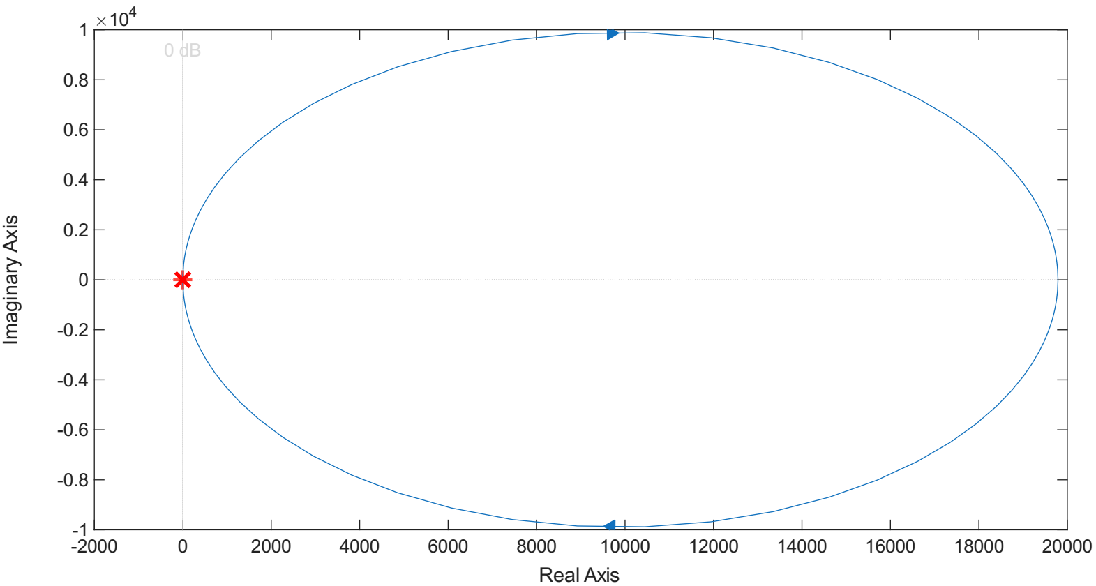
Diagrama de Nyquist distancia minima a -1 = 1/||S|| = 0.666
