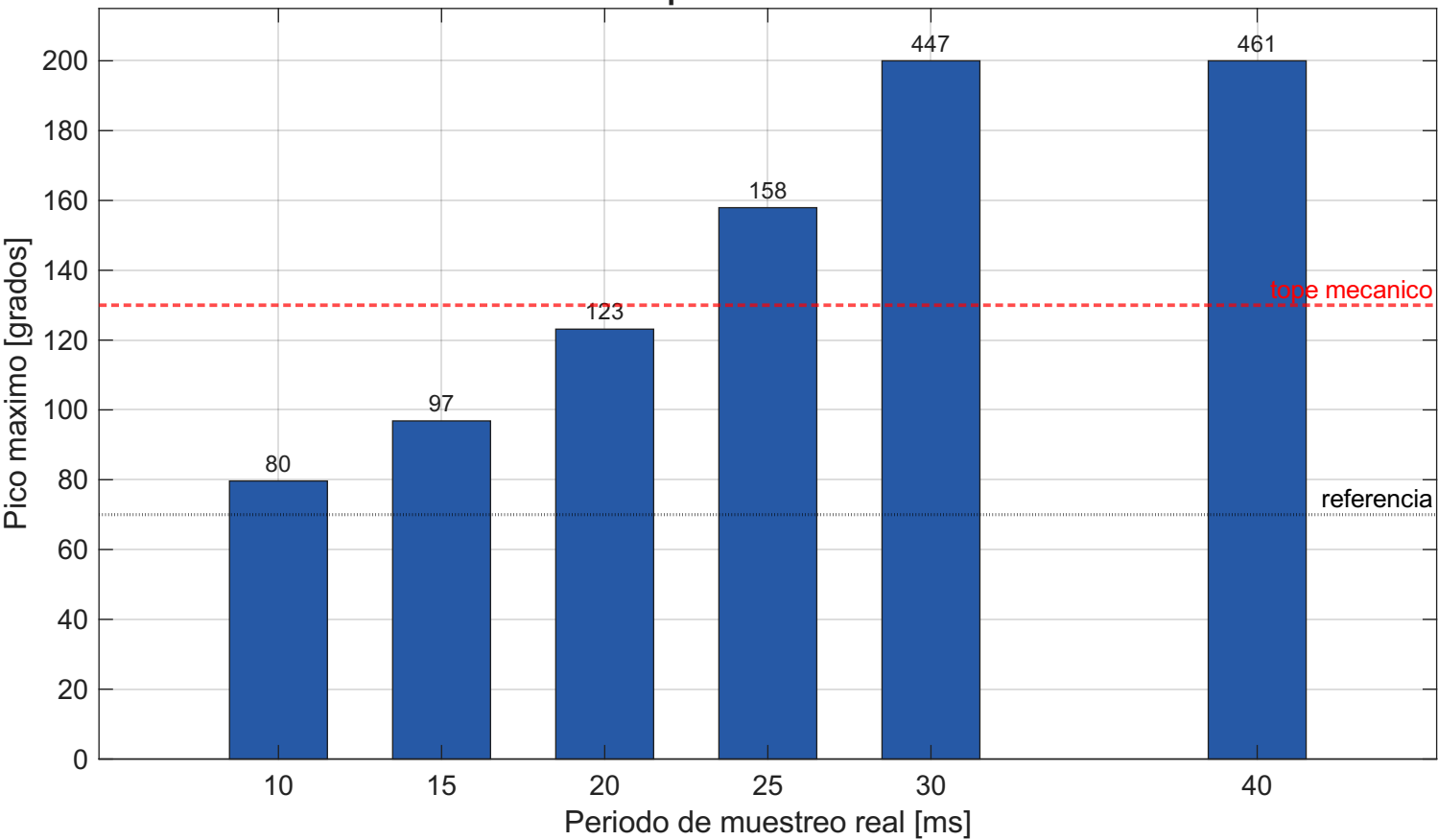
Sensibilidad al periodo de muestreo del lazo
