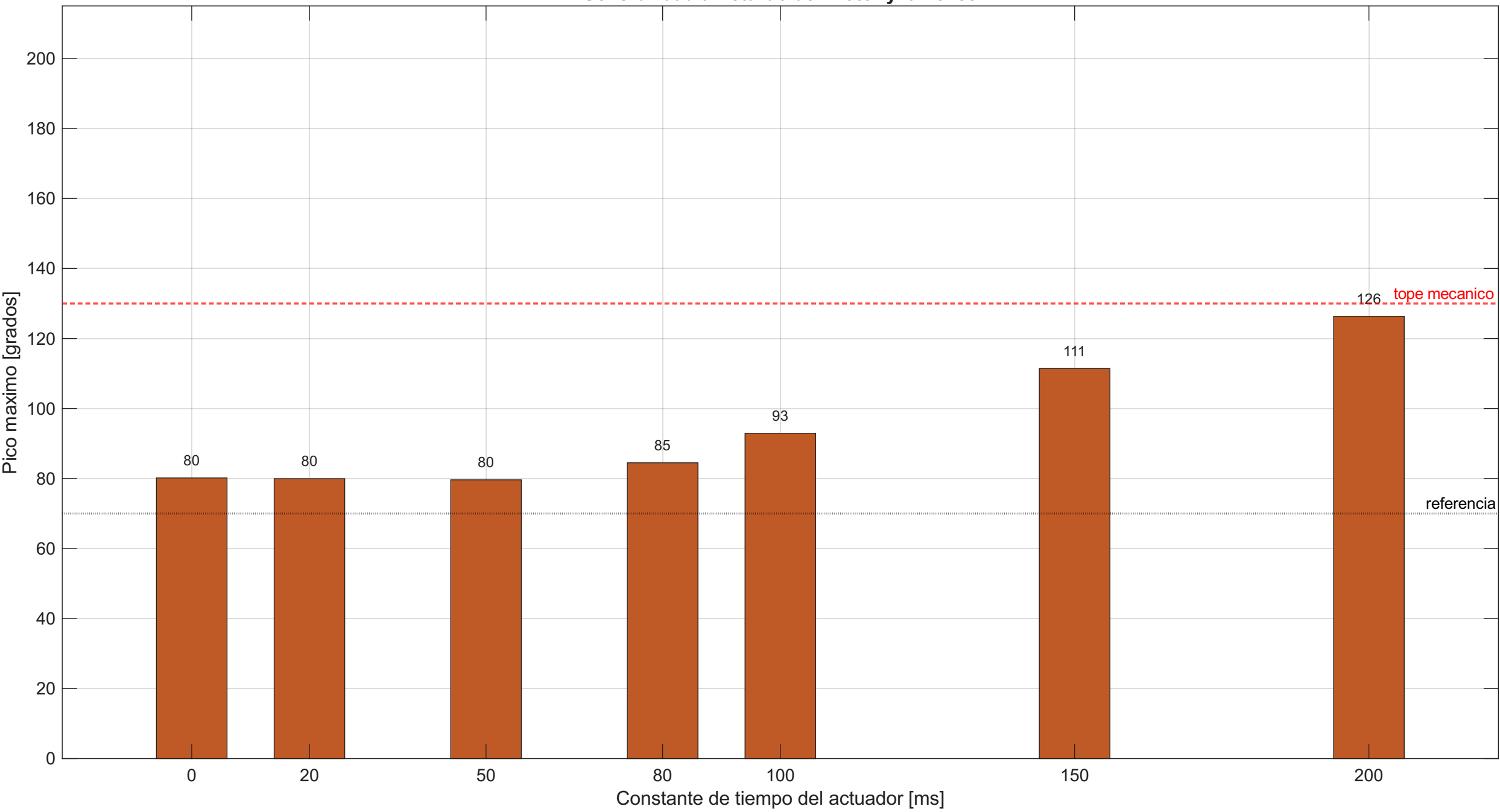
Sensibilidad al retardo del motor y la helice
