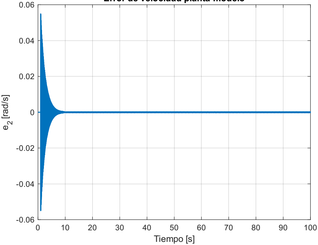
Error de velocidad planta-modelo
