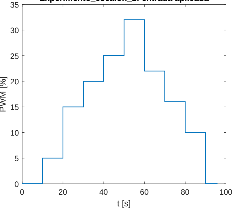
Experimento_escalon_1: entrada aplicada
