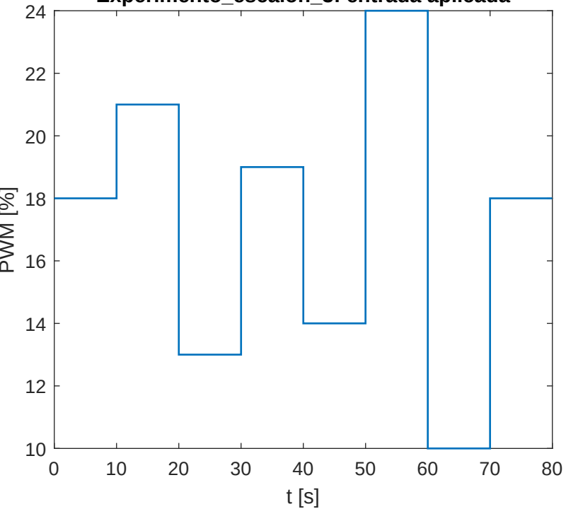
Experimento_escalon_3: entrada aplicada
