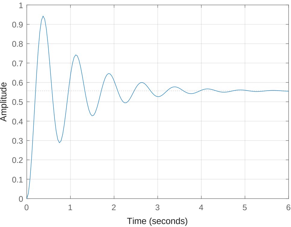
Respuesta con control P ( K_p = 0.28 )
