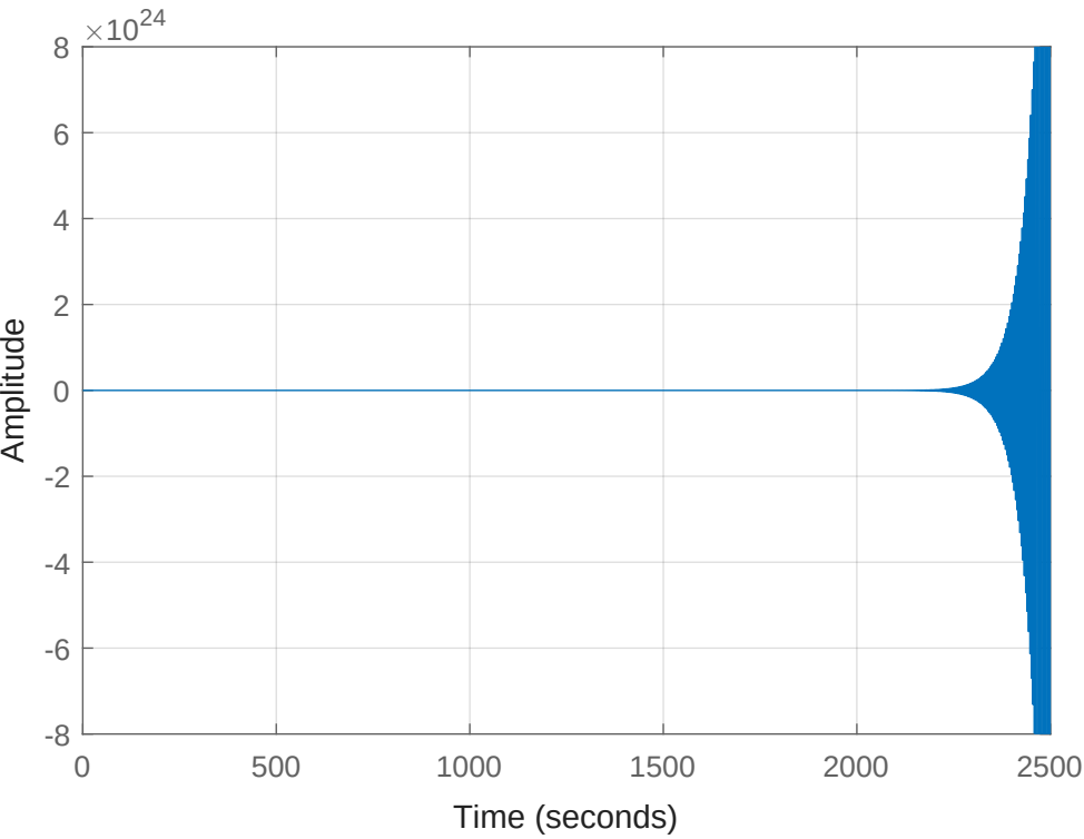
Respuesta con control PI ( K_p = 0.28 , K_i = 1.00 )
