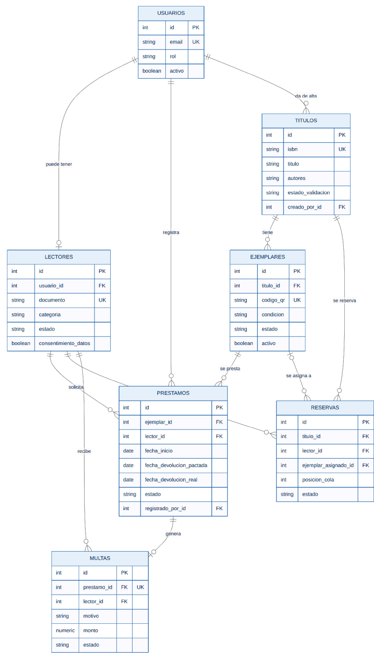
Figura 1 — Diagrama entidad-relación (ERD) — Base de datos
