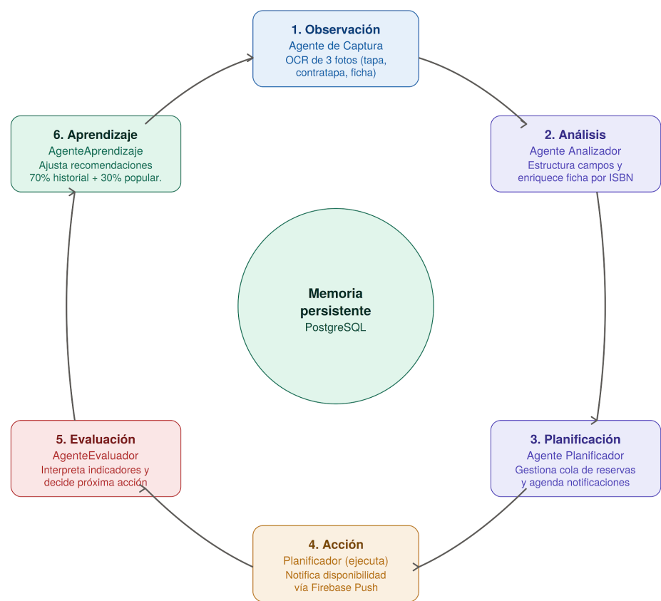
Figura 2 — Diagrama de flujo de agentes
