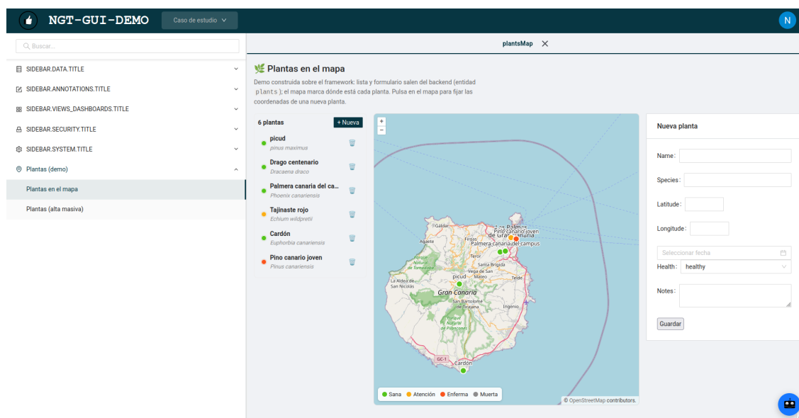
Ilustración 7.4: Demo «Plantas en el mapa»: lista, mapa y formulario de alta generado automáticamente desde el esquema de la entidad plants .
