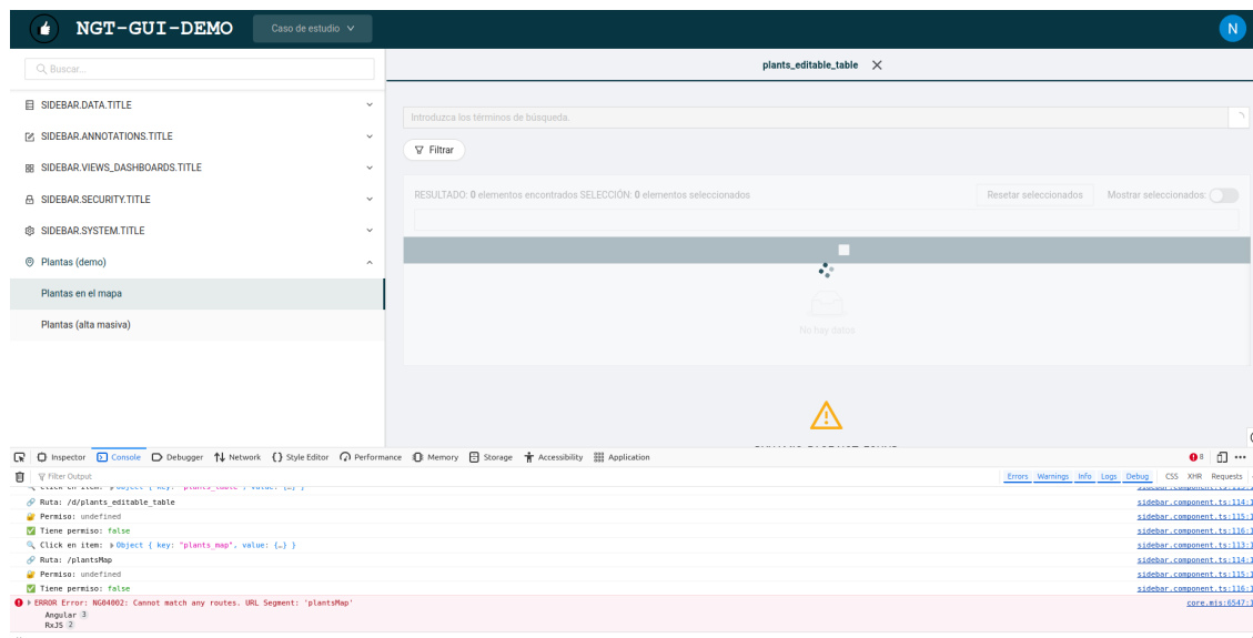
Ilustración 7.3: Generación dinámica de la interfaz: menú lateral y pantalla de entidad contruidos a partir del esquema.
