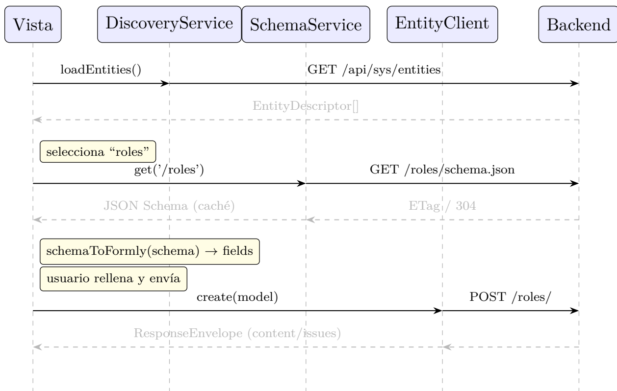
Ilustración 7.4: Secuencia de integración extremo a extremo.
