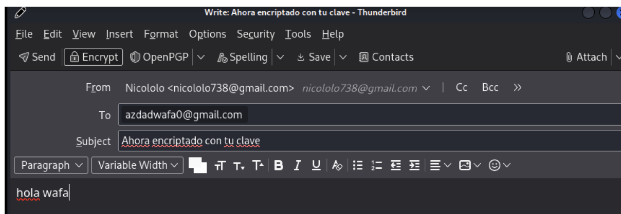
Figura 3.3: Composición del mensaje cifrado y firmado con OpenPGP dirigido a Wafa
