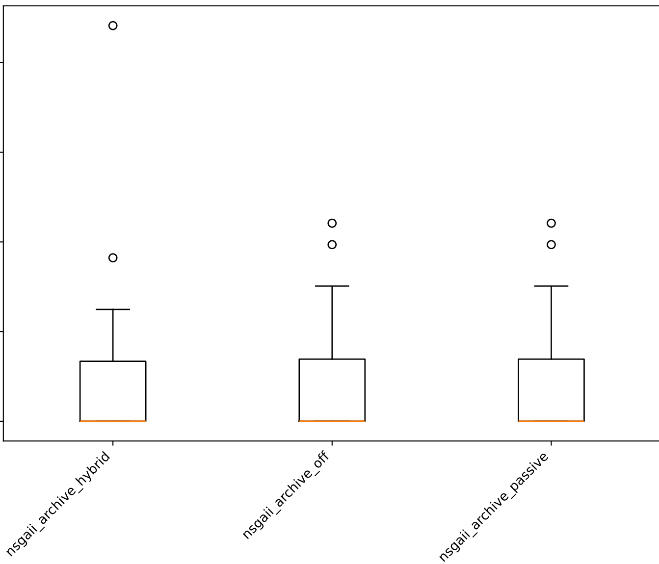
dtlz1
