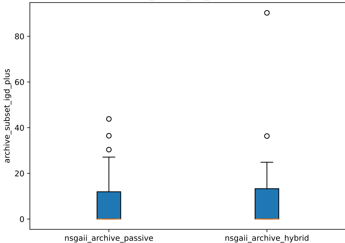
archive_subset_igd_plus | dtlz1
