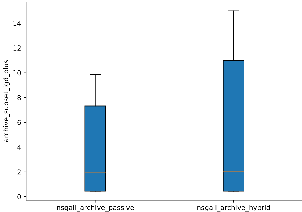
archive_subset_igd_plus | zcat10
