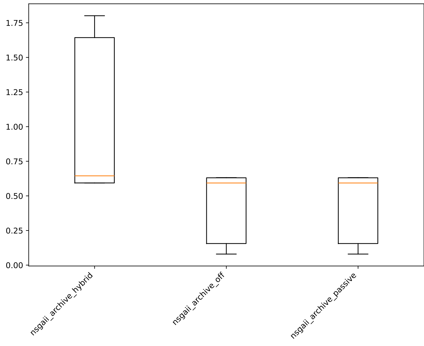
dtlz2
