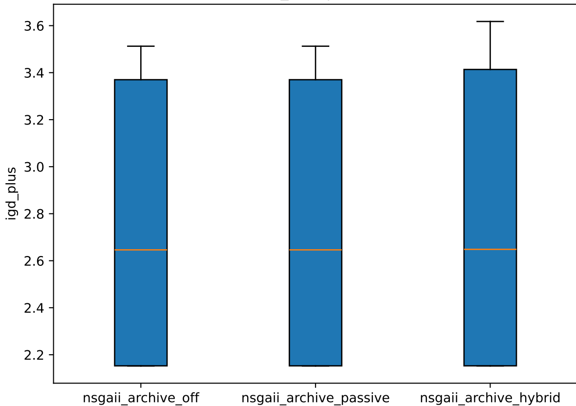
igd_plus | dtlz7
