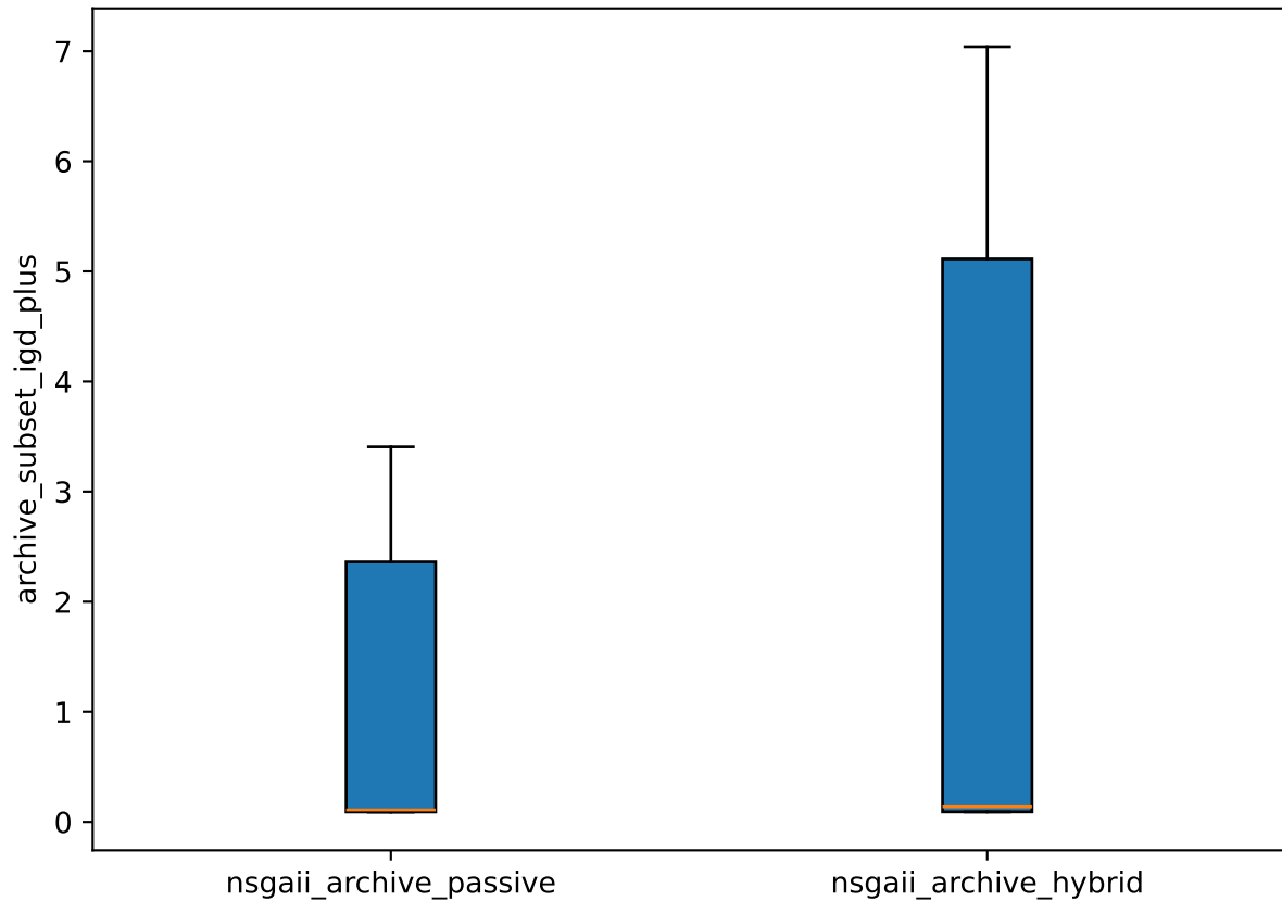
archive_subset_igd_plus | zcat1
