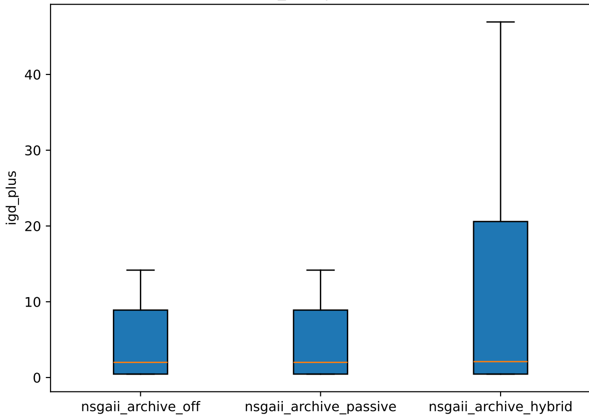
igd_plus | zcat10
