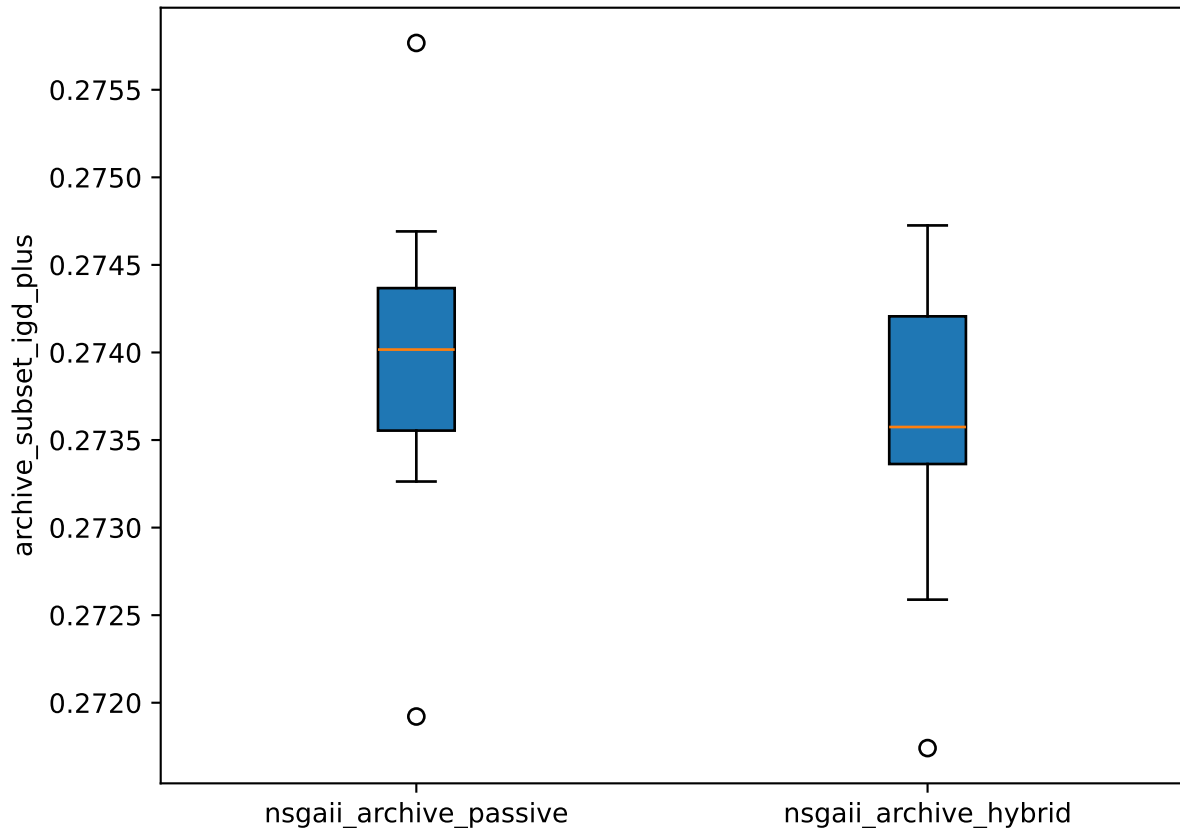
archive_subset_igd_plus | zdt1
