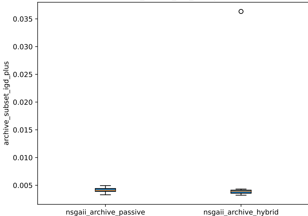
archive_subset_igd_plus | zdt3
