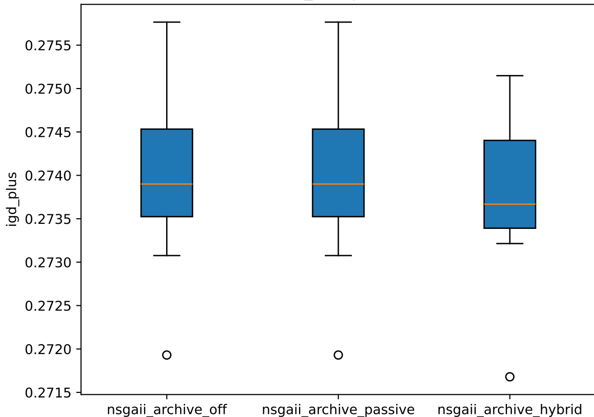
igd_plus | zdt1
