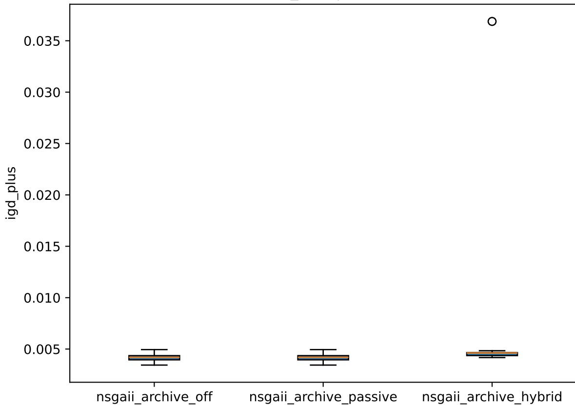
igd_plus | zdt3
