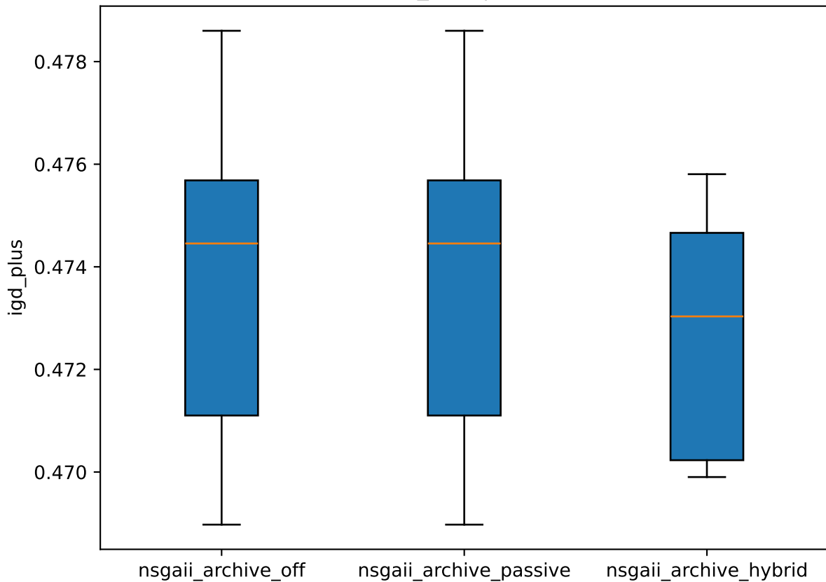
igd_plus | zdt6
