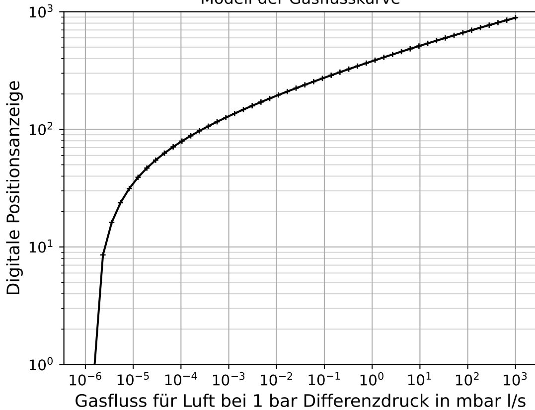
Modell der Gasflusskurve
