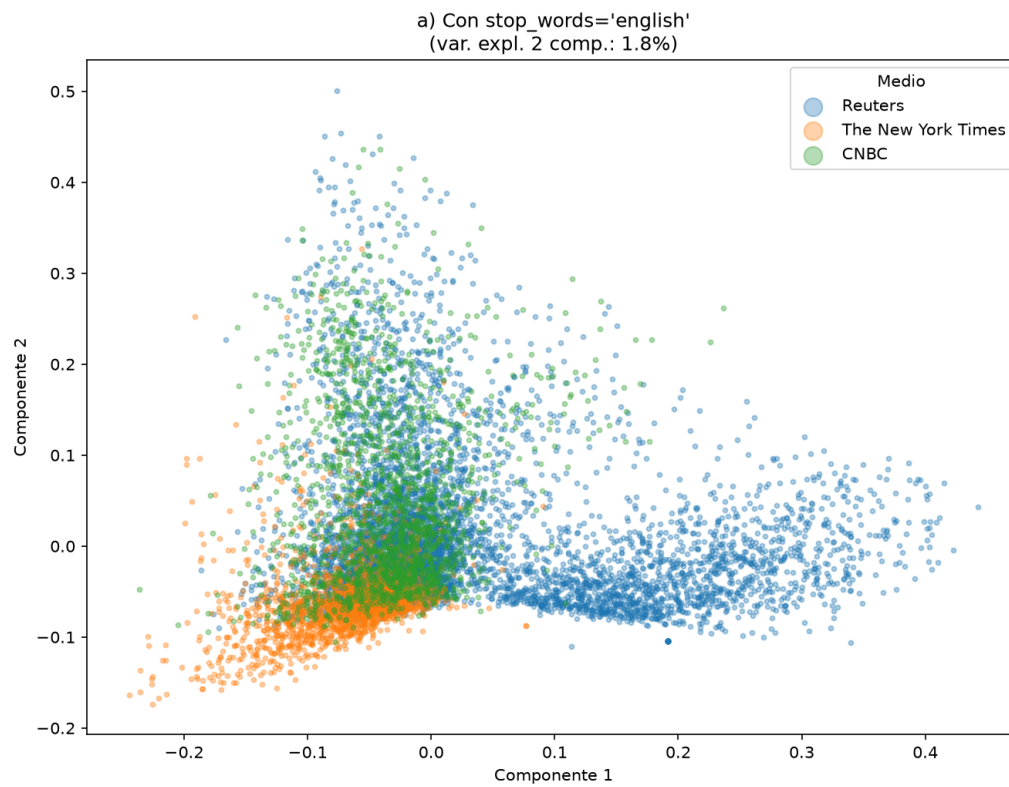
Figura 4: PCA con stop_words='english'.
