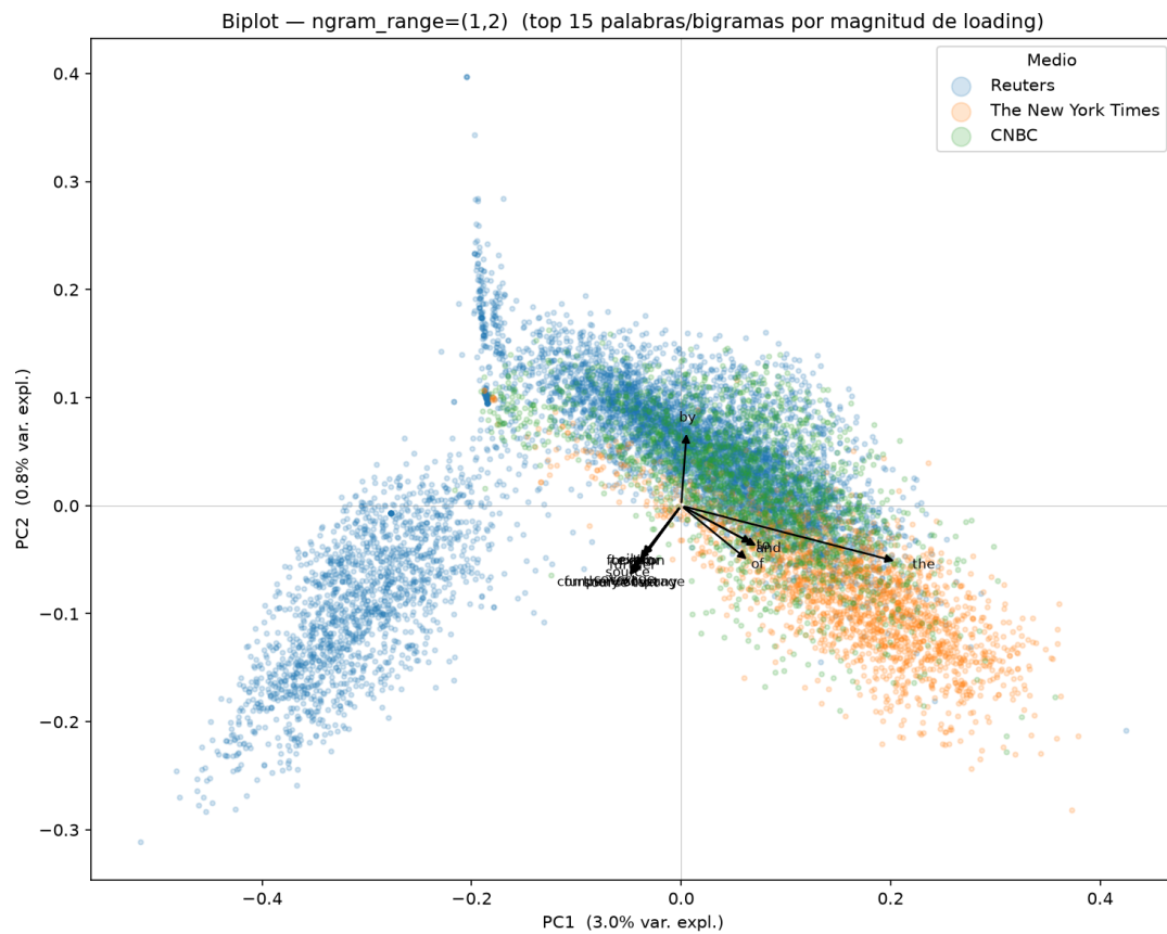
Figura 9: Biplot con bigramas: aparecen expresiones compuestas características de cada medio.
