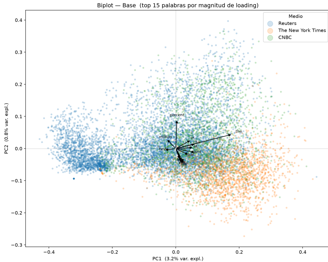
Figura 3: Biplot sobre TF-IDF base: puntos coloreados por medio y flechas con las 15 palabras de mayor loading.
