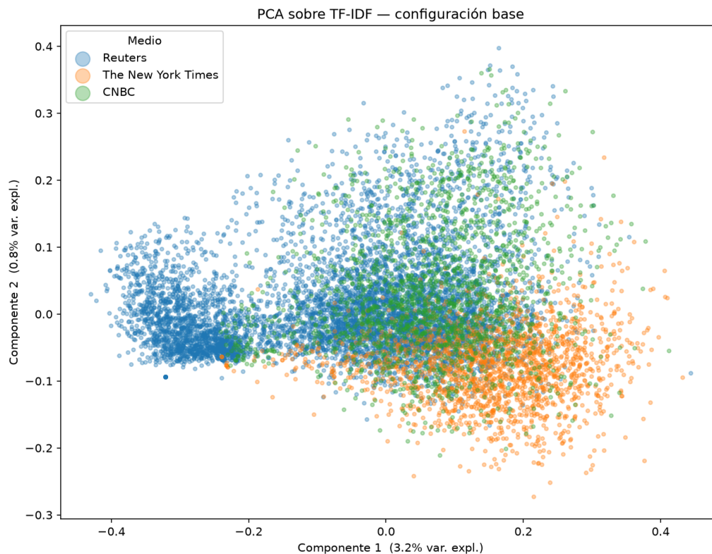
Figura 2: Mapa PCA (2 primeras componentes) sobre TF-IDF base, coloreado por medio de prensa.
