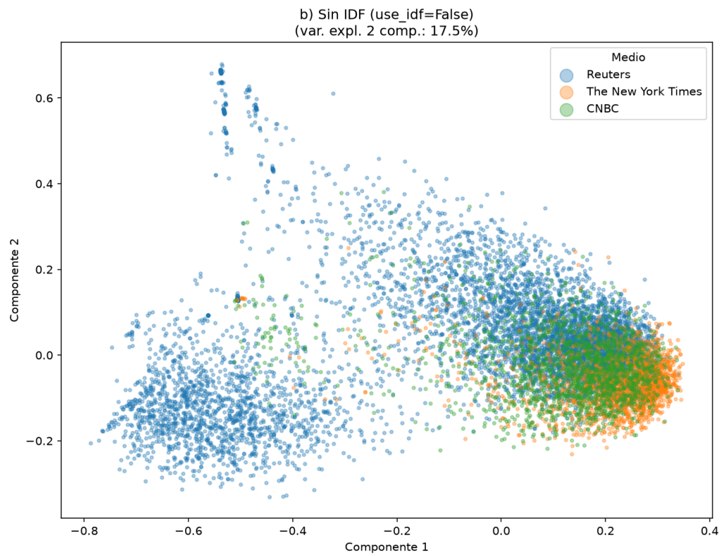
Figura 6: PCA con use_idf=False (TF puro).
