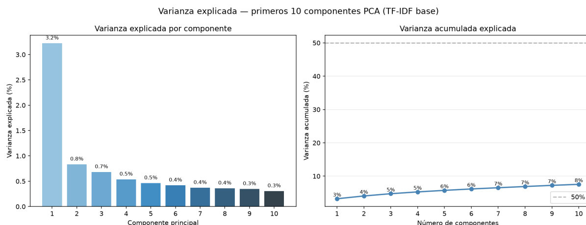
Figura 10: Varianza explicada por cada componente principal (izquierda) y varianza acumulada (derecha) para los primeros 10 componentes sobre la configuración TF-IDF base.
