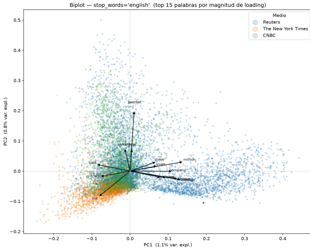
Figura 5: Biplot con stop_words='english' : al eliminar palabras funcionales, los loadings quedan dominados por términos de contenido.
