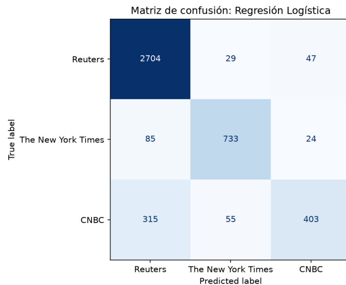
Figura 10: Matriz de confusión de la regresión logística sobre el conjunto de test.
