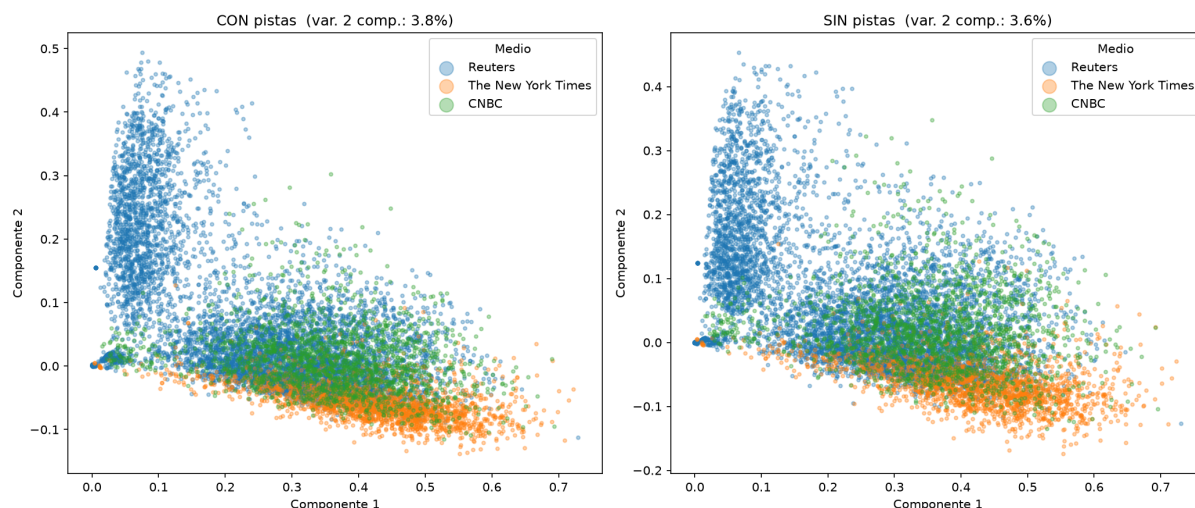
Figura 14: Mapas de 2 componentes (TruncatedSVD) con (izquierda) y sin (derecha) las pistas del medio. La estructura es prácticamente idéntica: Reuters sigue separándose con claridad y NYT/CNBC se mantienen superpuestos, lo que confirma que la separación observada en la Parte 1 es genuína y no un artefacto del boilerplate .
