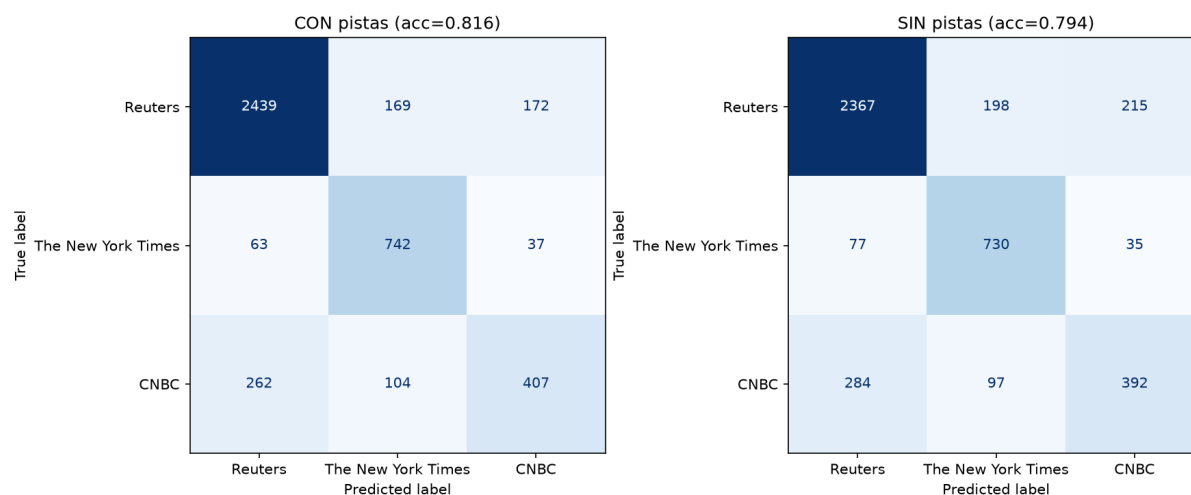
Figura 13: Matrices de confusión del MNB con (izquierda) y sin (derecha) las pistas del medio. Al remover las pistas, Reuters pierde aciertos (de 2.439 a 2.367) que pasan a confundirse con los otros dos medios, pero el efecto es moderado.
