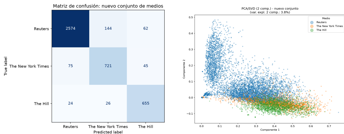
Figura 12: Izquierda: matriz de confusión del MNB sobre el nuevo conjunto. Derecha: mapa de 2 componentes (TruncatedSVD) del nuevo conjunto de entrenamiento.
