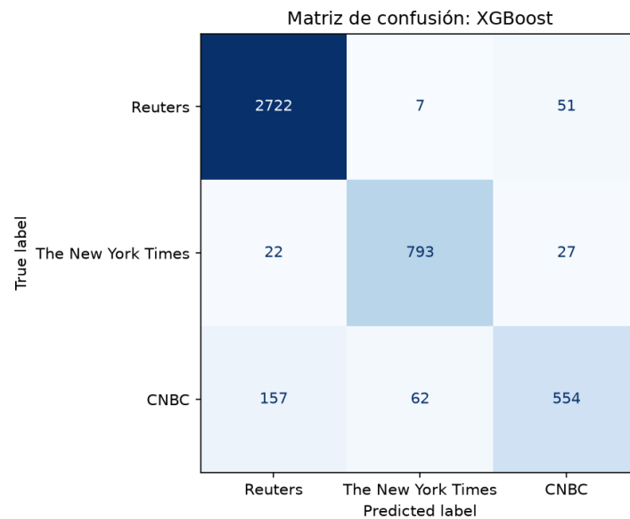
Figura 11: Matriz de confusión de XGBoost sobre el conjunto de test.
