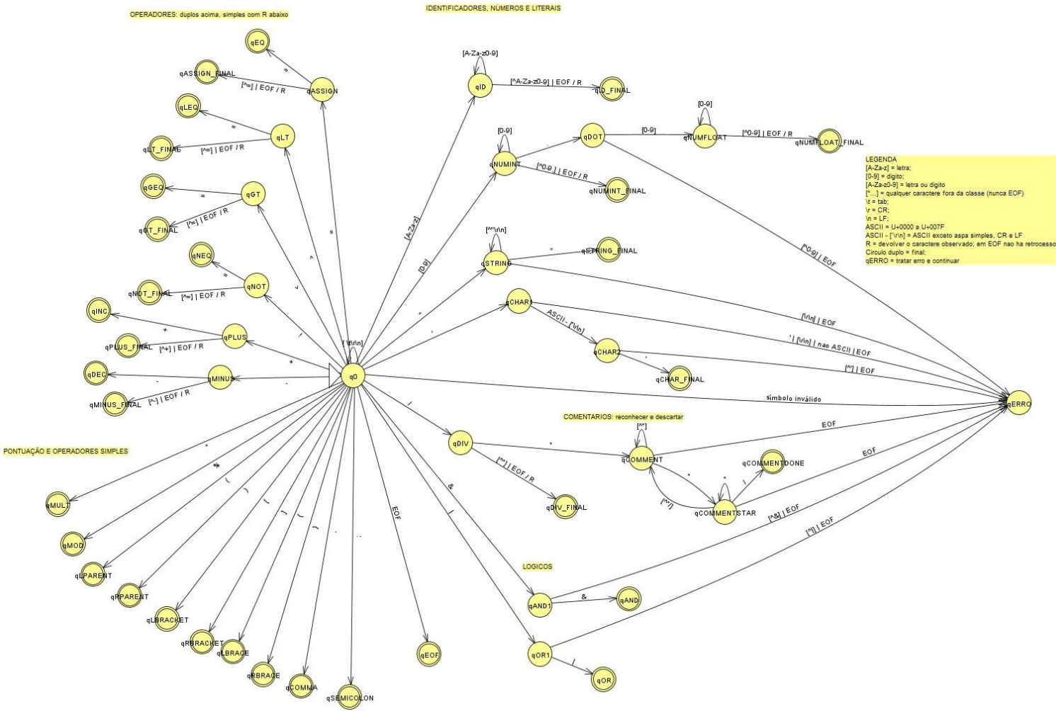
Figura 1: AFD projetado para o analisador léxico de C--.
