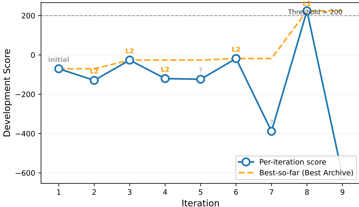
Score Trajectory — CREATE seed_0 (LunarLander-v3)
