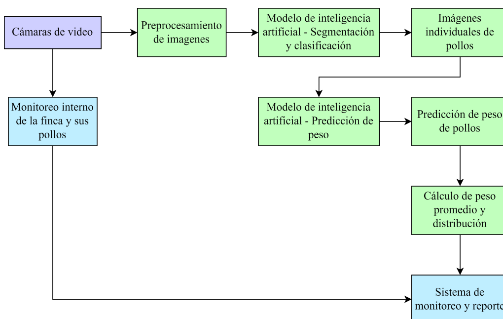
Figura 4. Diagrama en bloques del sistema.
