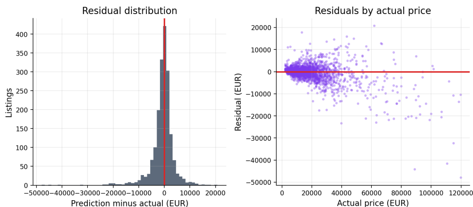
Figura 9.4: Analiza reziduurilor pentru modelul ales
