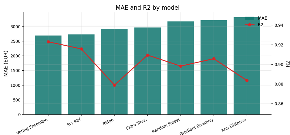
Figura 9.2: MAE și R^2 pentru modelele evaluate
