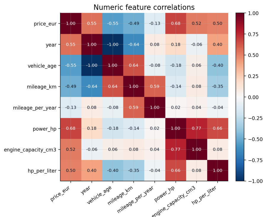
Figura 9.5: Matrice de corelații pentru caracteristici numerice
