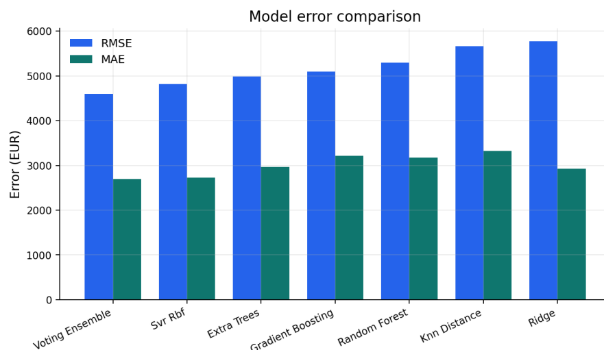
Figura 9.1: Comparație de performanță între modele
