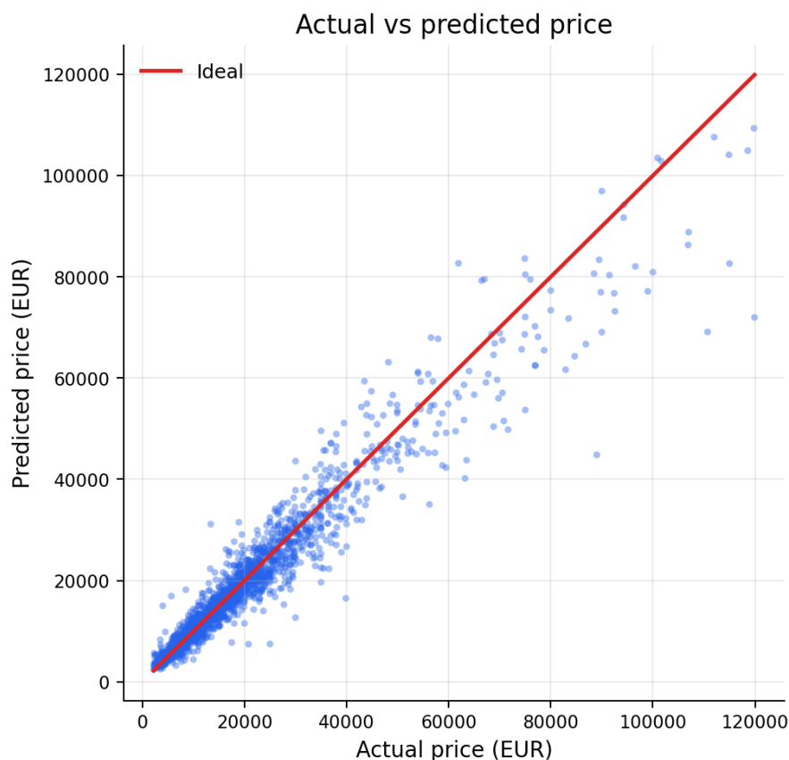
Figura 9.3: Preț real față de preț estimat
