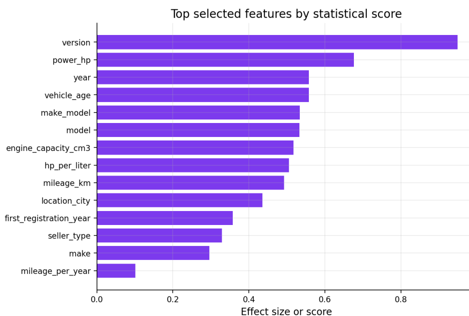
Figura 6.1: Caracteristici relevante după testele statistice
