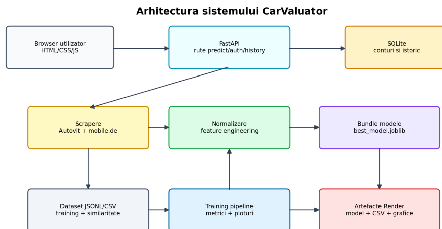
Figura 7.1: Arhitectura sistemului CarValuator
