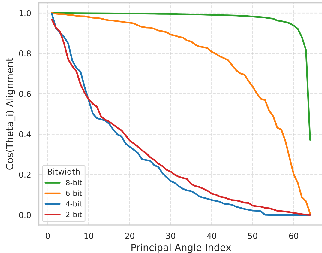
Per-Tensor (k=64)
