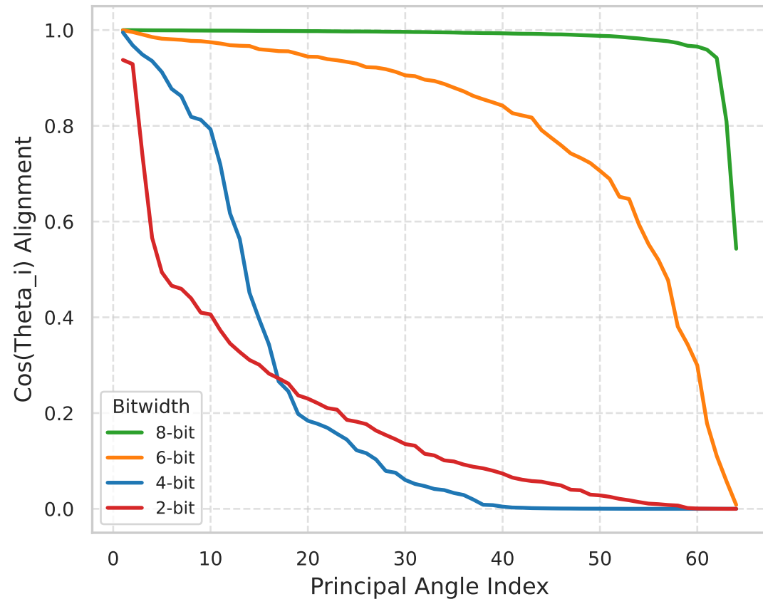
Per-Tensor (k=64)
