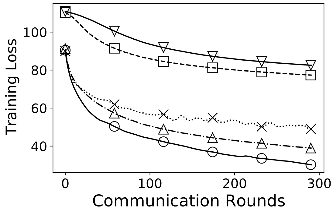
CIFAR10
