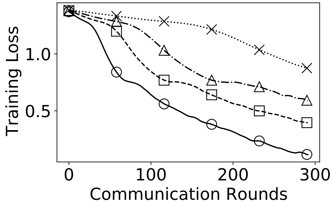
CREMA-D
