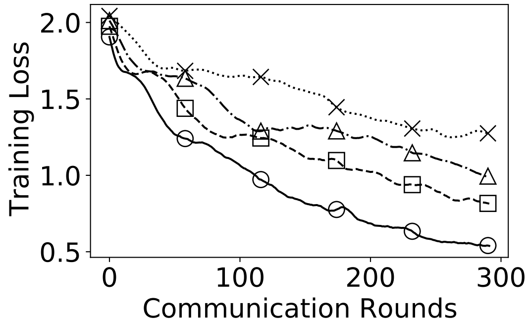
KU-HAR
