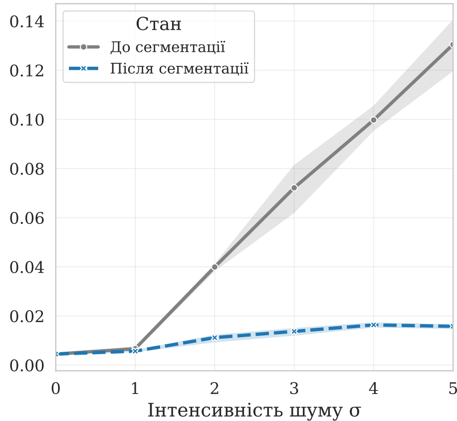
Велика мережа (~950 пристроїв)
